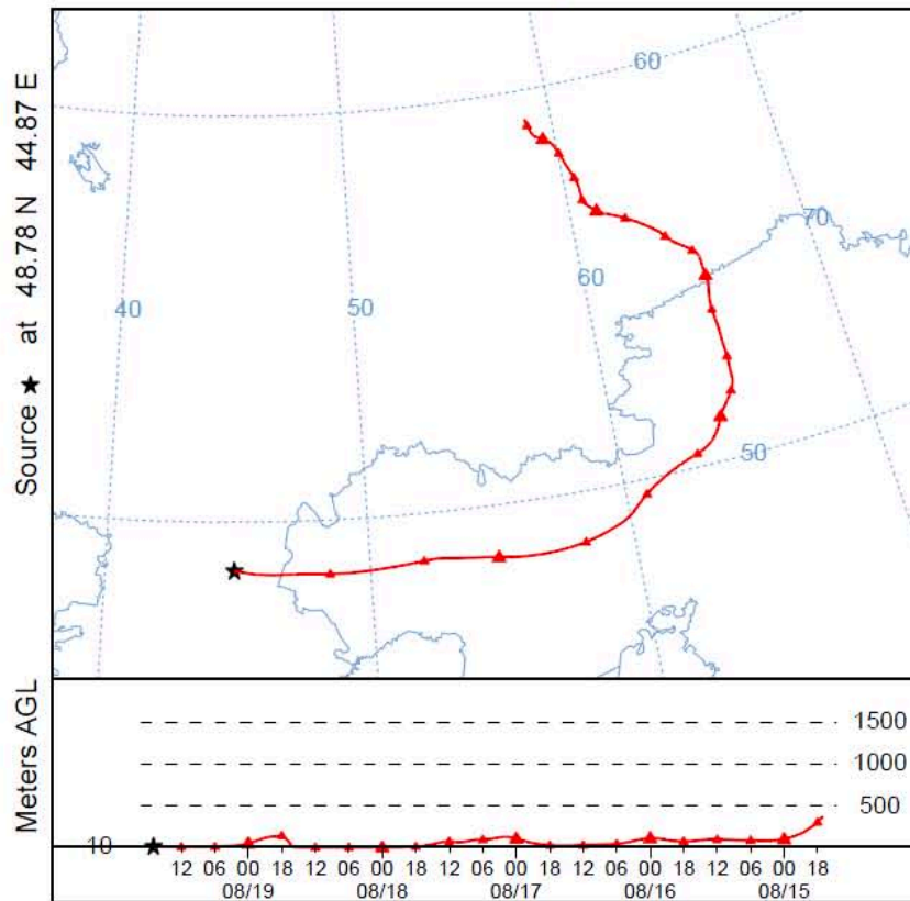
Рисунок 3: Обратная траектория аэрозолей для г. Волжский на высоте 10 м, с датой начала 15 августа 2022 г.
